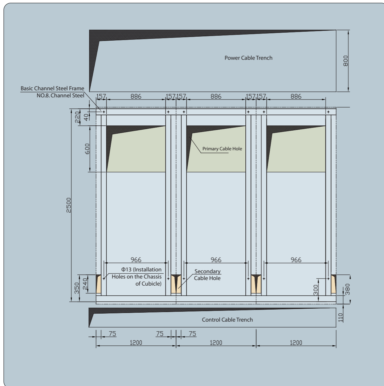
离墙安装开关柜的基础宽架的结构示意图
