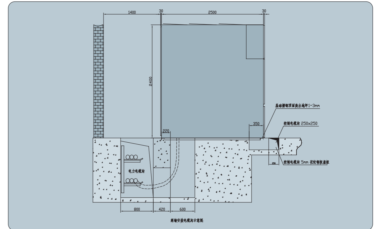
离墙安装电缆沟示意图
