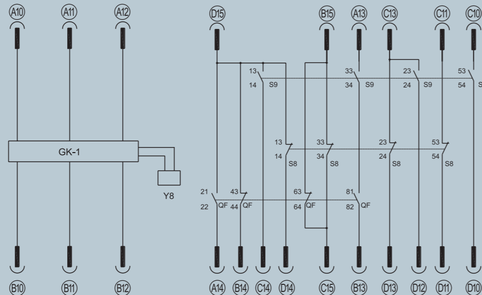
过流脱扣(A相) 过流脱扣(C相) 过流脱扣(B相)
