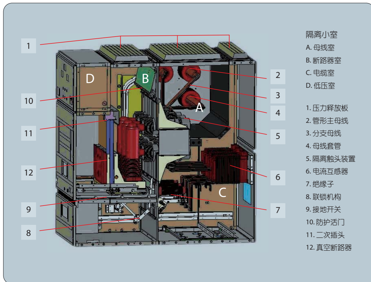
ZSG-40.5开关柜内部结构图
